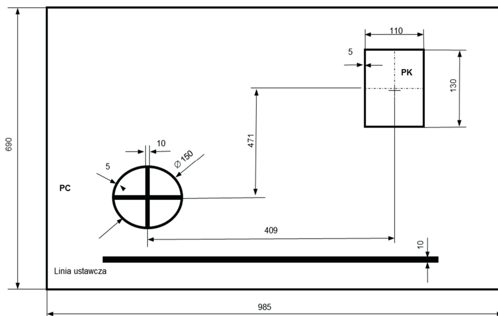
Rysunek 2-32. Tarcza do przystrzeliwania sprzężonego km PKT BWP-1.
