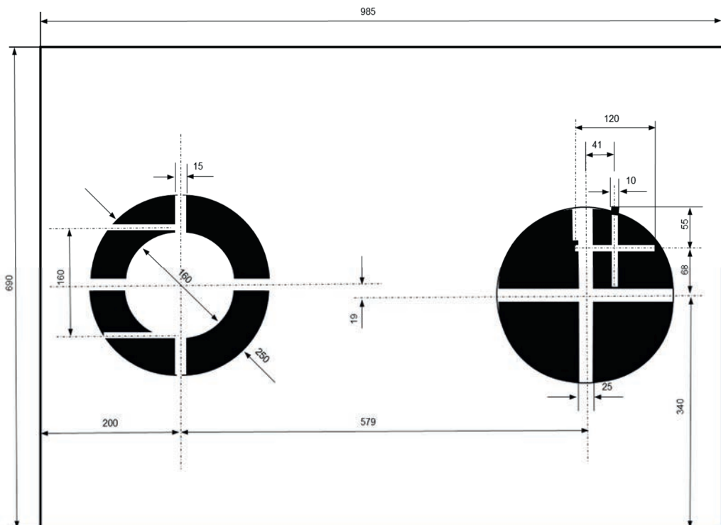
Rysunek 2-43. Tarcza współrzędnych do zgrywania przyrządów celowniczych rgppanc-7.
