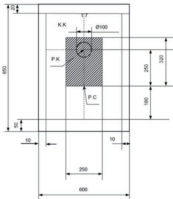
Rysunek 2-22. Tarcza do przystrzeliwania 5,56 mm karabinu szturmowego BERYL (100 m).
