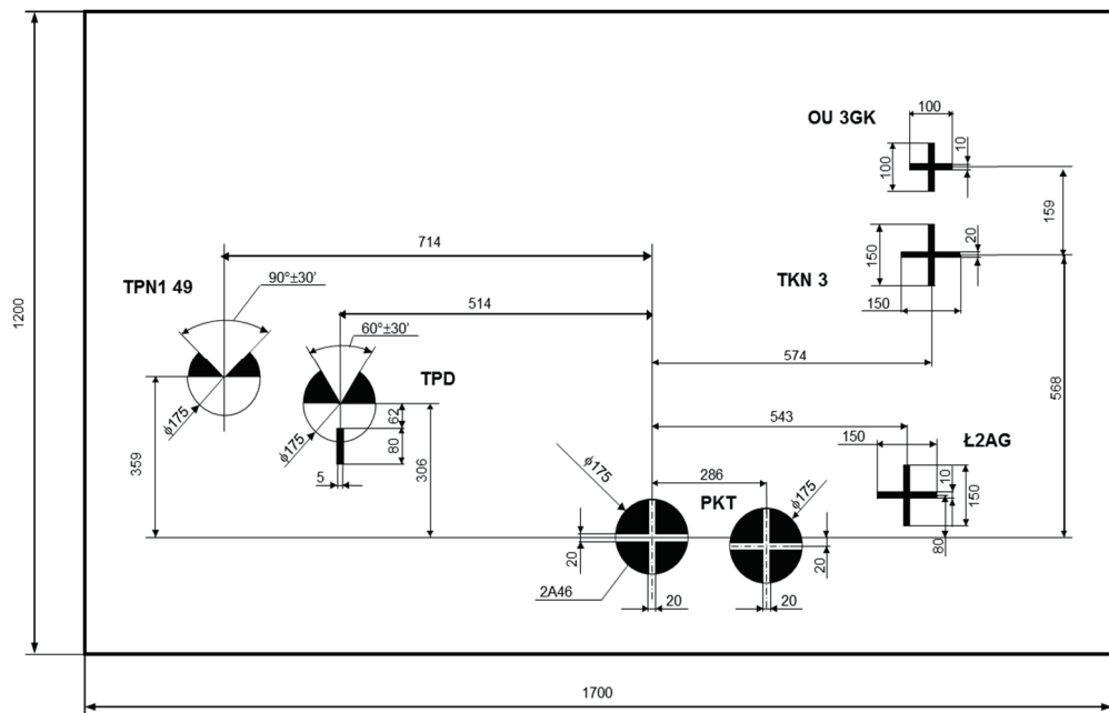
Rysunek 2-41. Tarcza współrzędnych do zgrywania uzbrojenia pokładowego T-72 (25 m).
